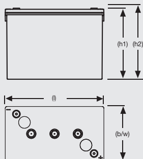
XL6V180
