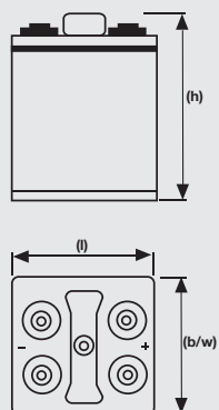
L2V320 - L2V425
