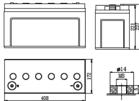
Выход В-M8
