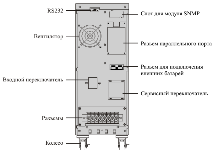
(Тыловая панель ИБП 6 кВА)
