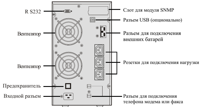
(Тыловая панель ИБП 2 кВА ~ 3 кВА)
