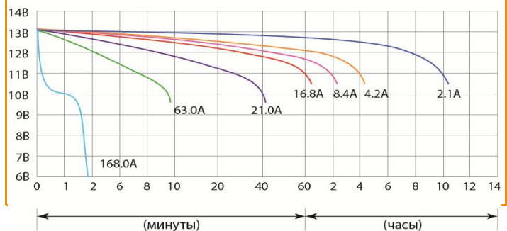
Разрядные характеристики (25°C)
