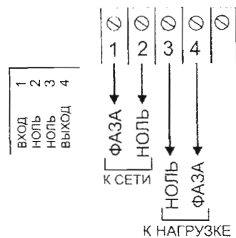
Рис.3. Подключение стабилизатора к сети и к нагрузке
