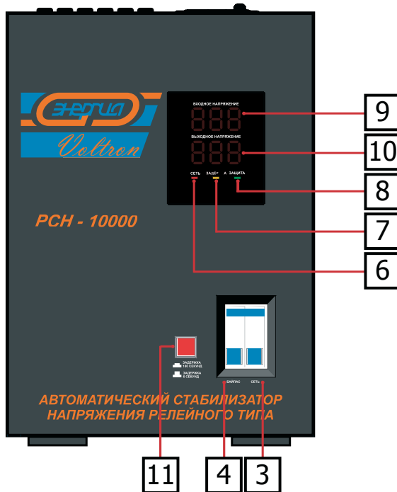
Лицевая панель
