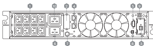
Вид сзади: KU9103S-RT (3 кВА)
