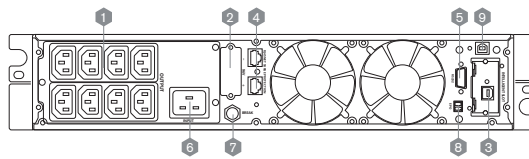
Вид сзади: KU9102S-RT (2 кВА)
