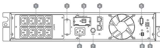
Вид сзади: KU9101S-RT (1 кВА)
