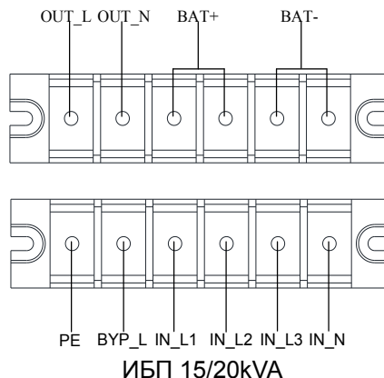
Рисунок 2-1: Схемы клеммных терминалов
