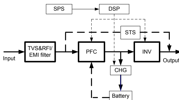
Рисунок 1-3: Структура ИБП
