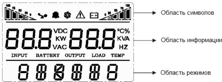
Рисунок 3-2: LCD дисплей
