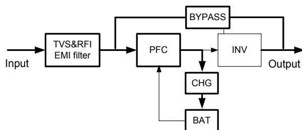
Рисунок 1-5: Режим байпаса
