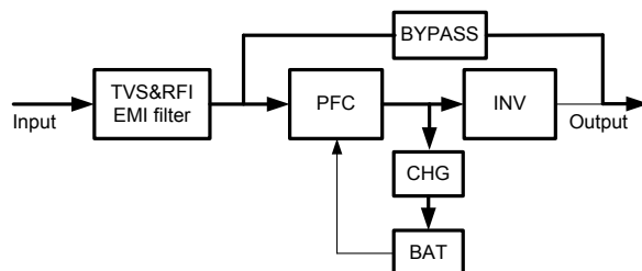
Рисунок 1-7: Режим ECO
