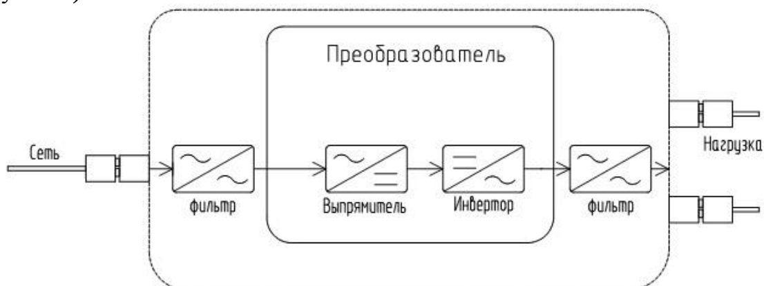
Рисунок 2 - Структурная схема принципа работы стабилизатора
