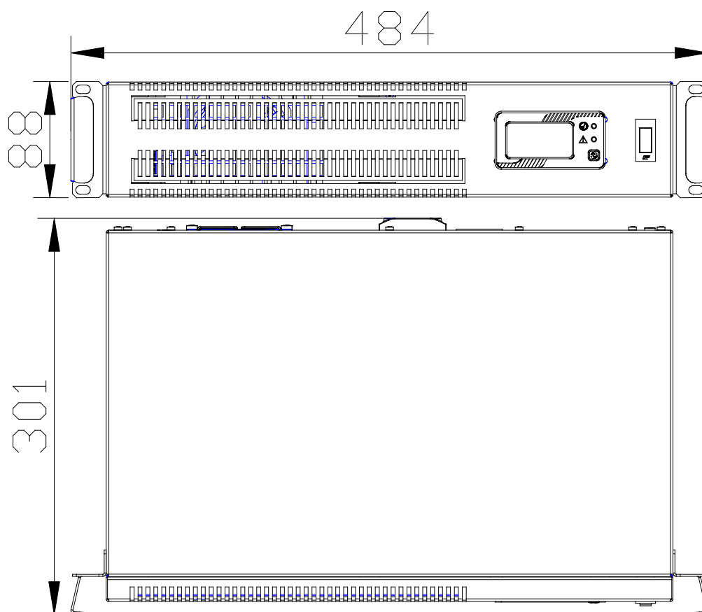
а) ИнСтаб IS1000R; ИнСтаб IS1500R
