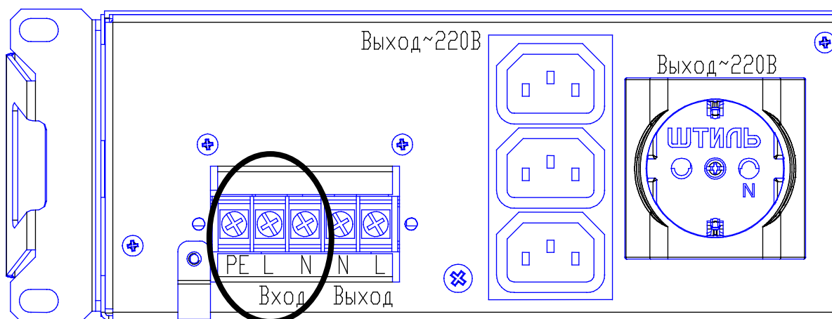
Рисунок 3.2 – Стабилизатор ИнСтаб. Клеммная колодка «Вход РЕ-L-N»
