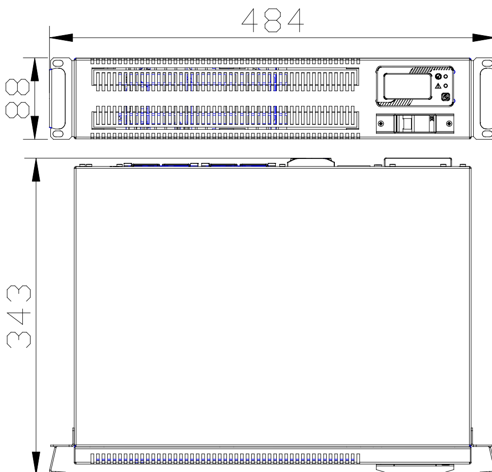
б) ИнСтаб IS2500R, ИнСтаб IS3500R
