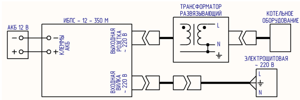
Рисунок 1 – Схема подключения ИБПС – 12 – 350 М
