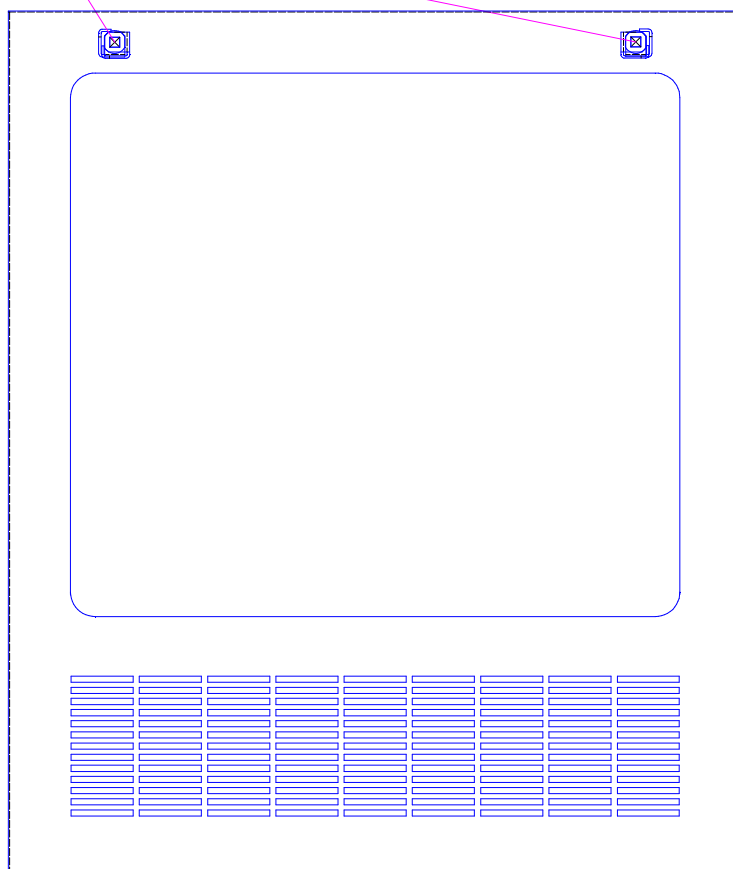
Рисунок 4.4 – Крепление замков на передней стенке.
