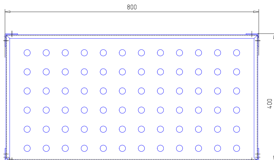
Рисунок 3.6 – Батарейный стеллаж Штиль MBS-03. Полка
