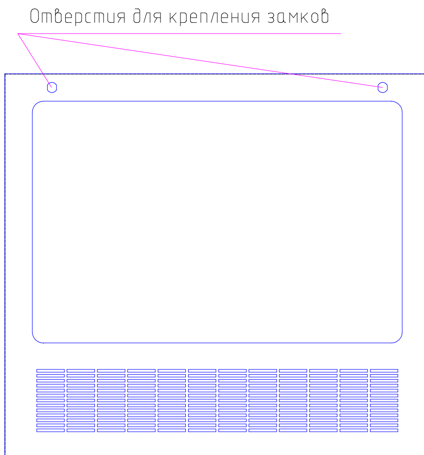
Рисунок 4.4 – Крепление замков на передней стенке.
