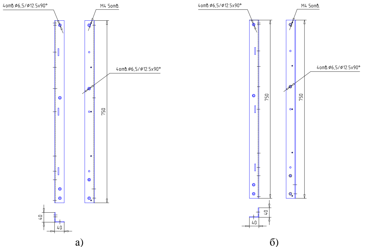
а) б) Рисунок 3.3 – Батарейный стеллаж Штиль МBS-04. а) - стойка передняя левая, б) - стойка передняя правая
